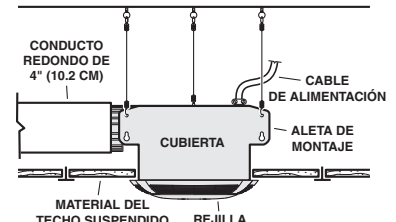
TECHOS SUSPENDIDOS Cubierta montada con cables. Montaje de tres puntos.
